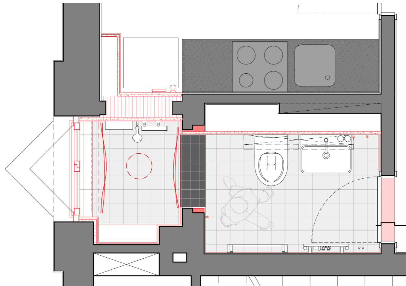
Grundriss Typ Loggia
