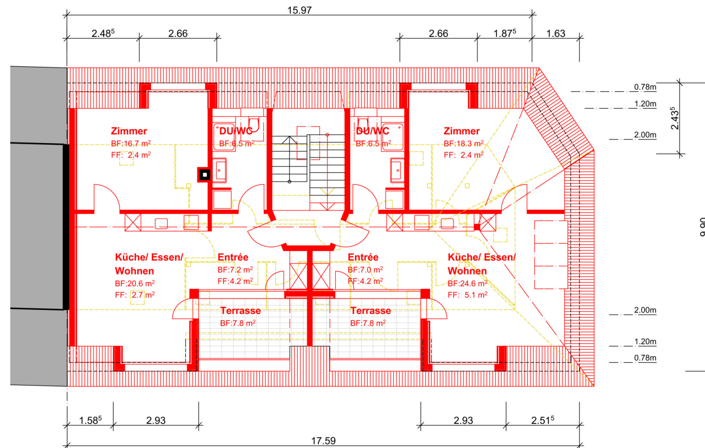
Grundriss
