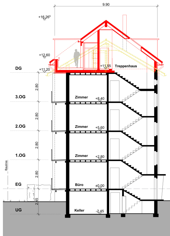
Schnitt
