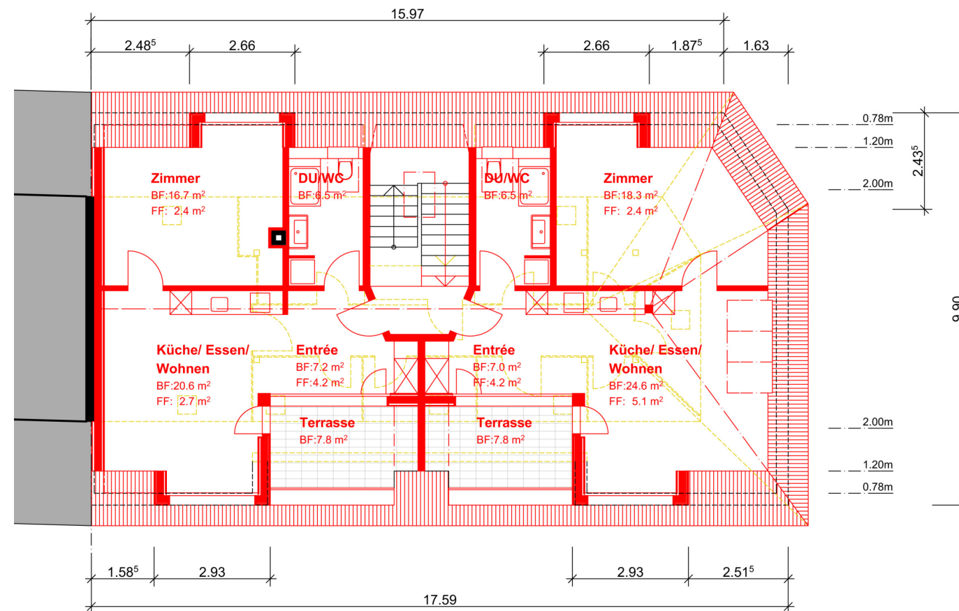
Grundriss
