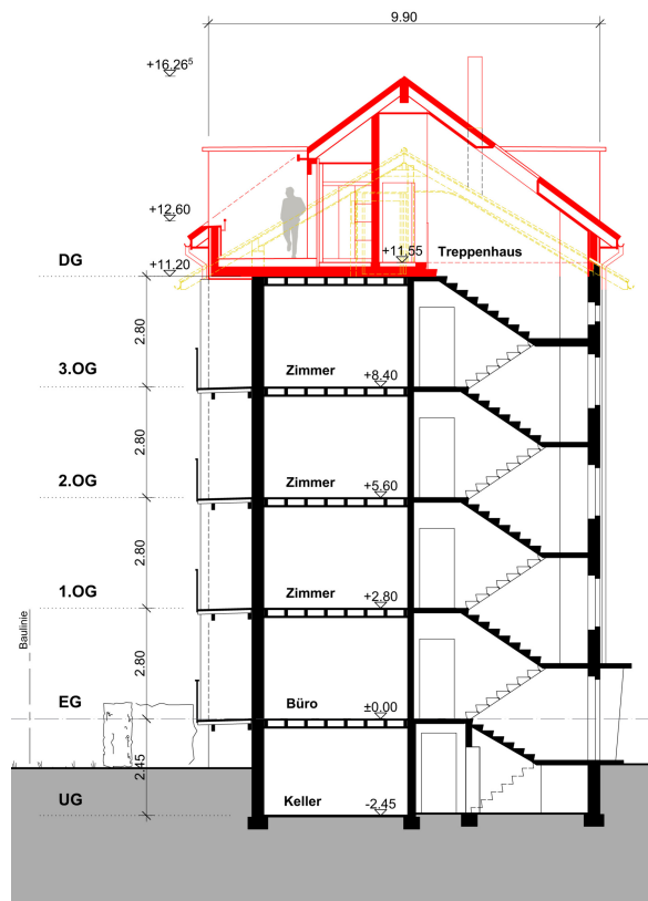
Schnitt
