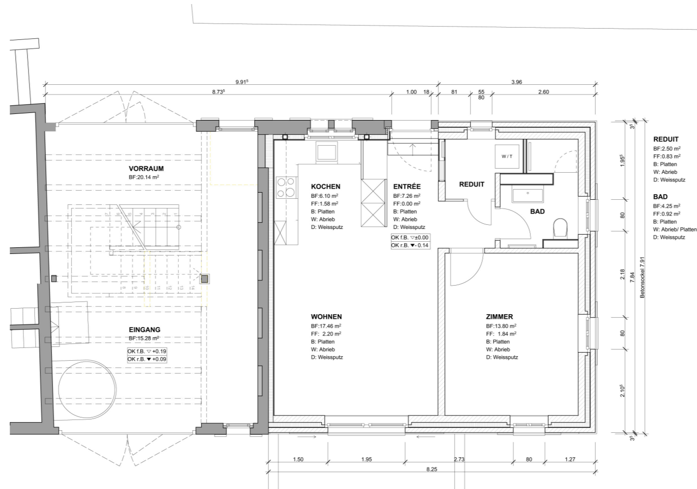
Grundriss Erdgeschoss
