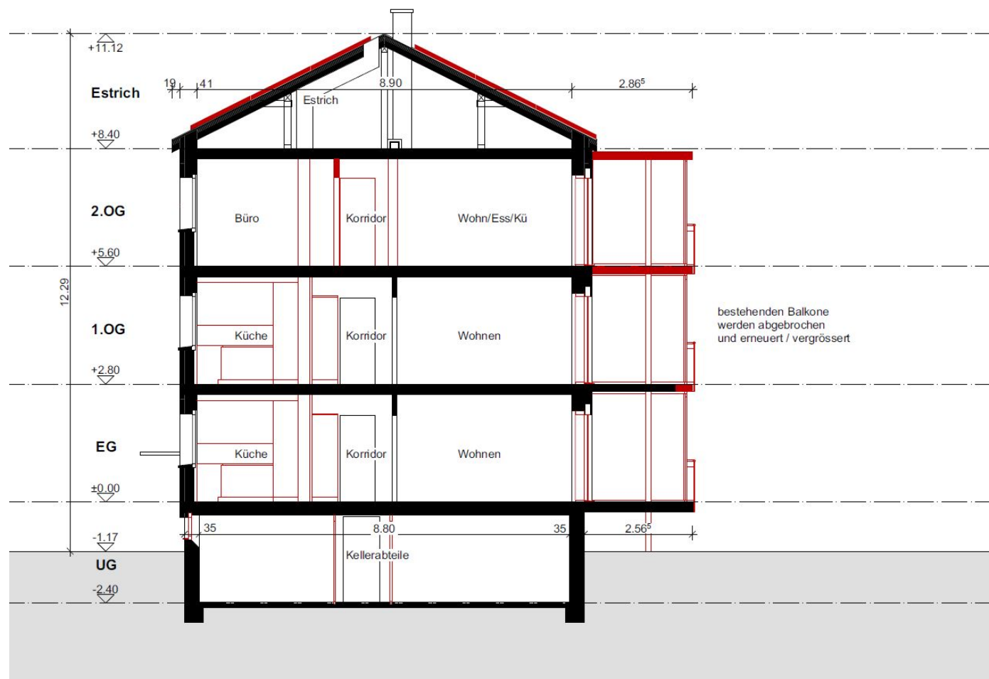
Querschnitt
