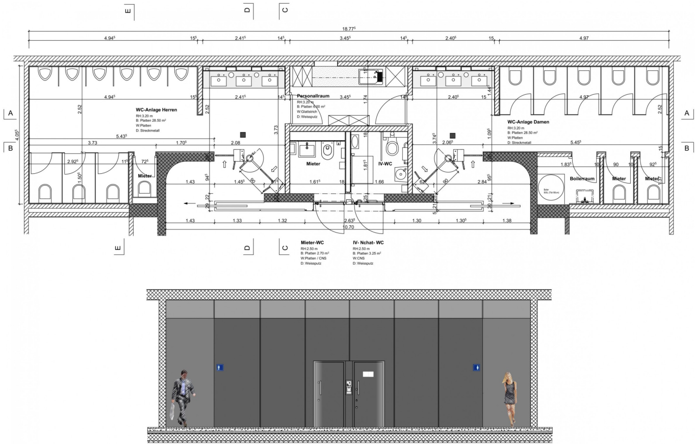
Grundriss neu/ Ansicht Aussenfront
