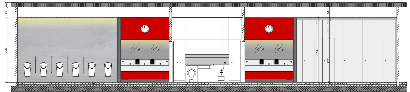
Ansicht A
