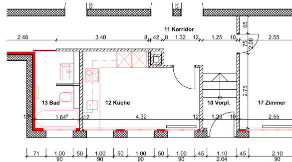
Wohnung 1
