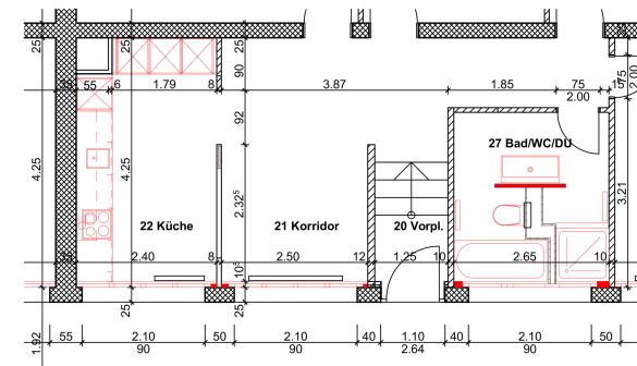
Wohnung 2
