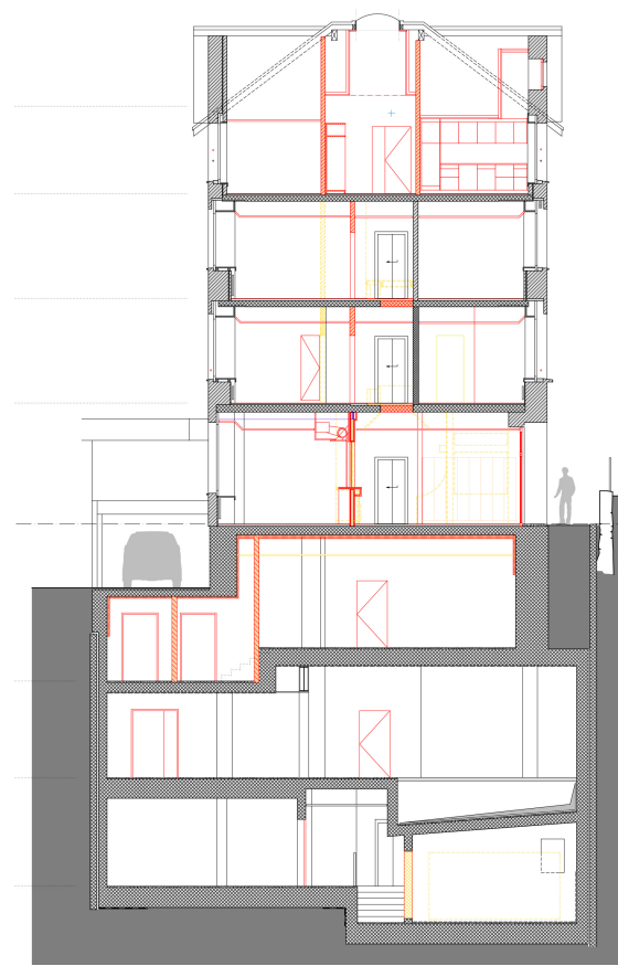
Gebäudeschnitt
