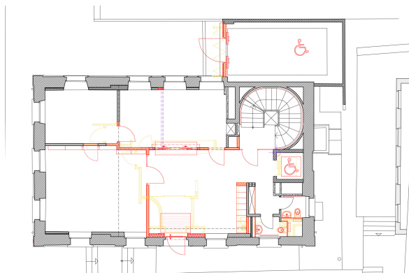
Grundriss Erdgeschoss
