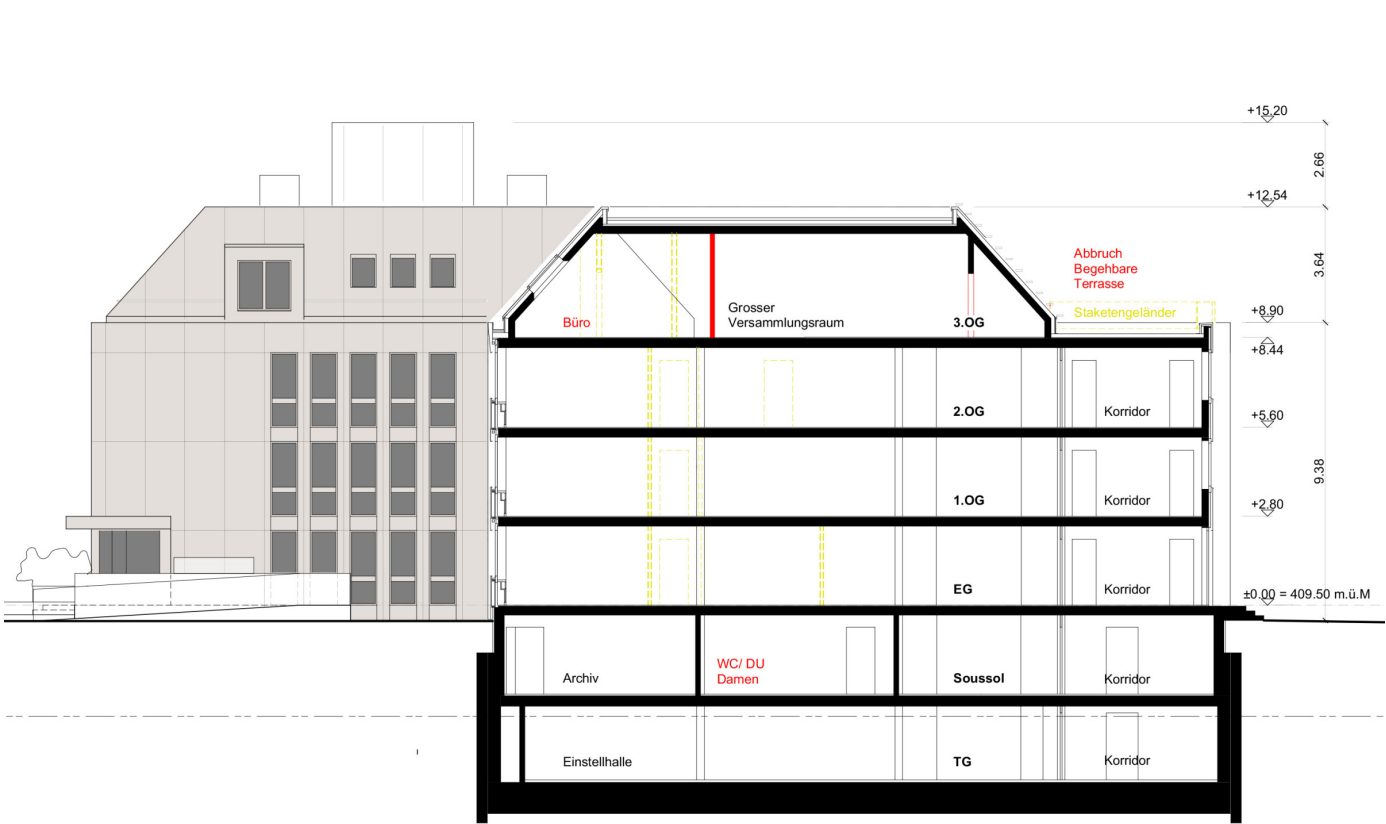
Gebäudeschnitt
